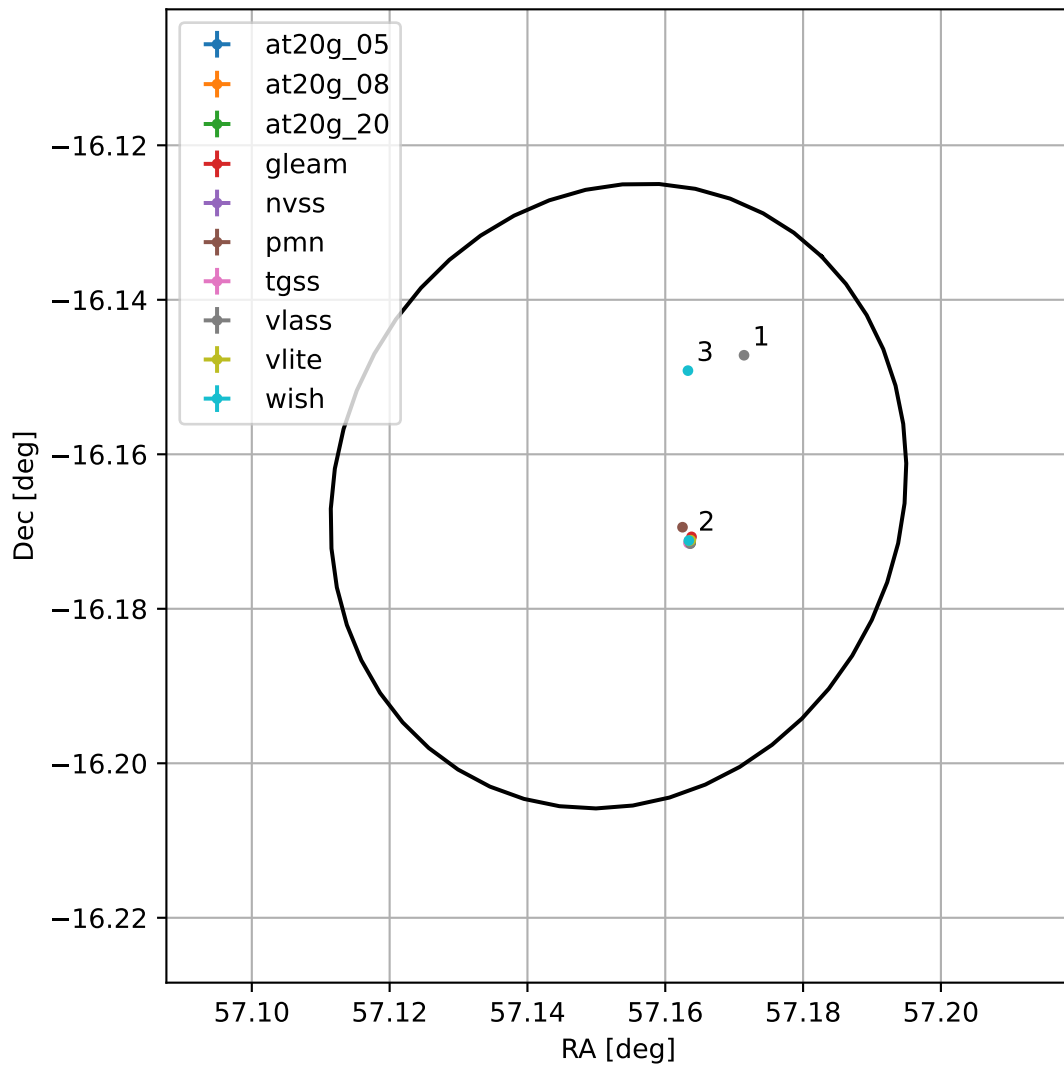
4FGL J0348.6-1609
