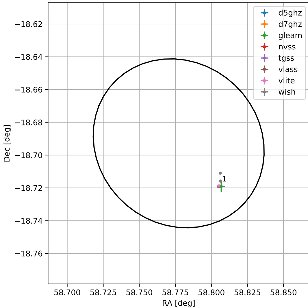
4FGL J0355.1-1841
