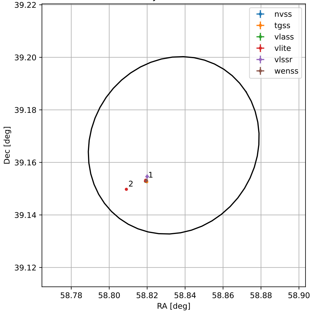
4FGL J0355.3+3909
