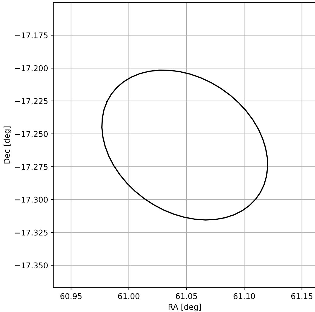
4FGL J0404.1-1715
