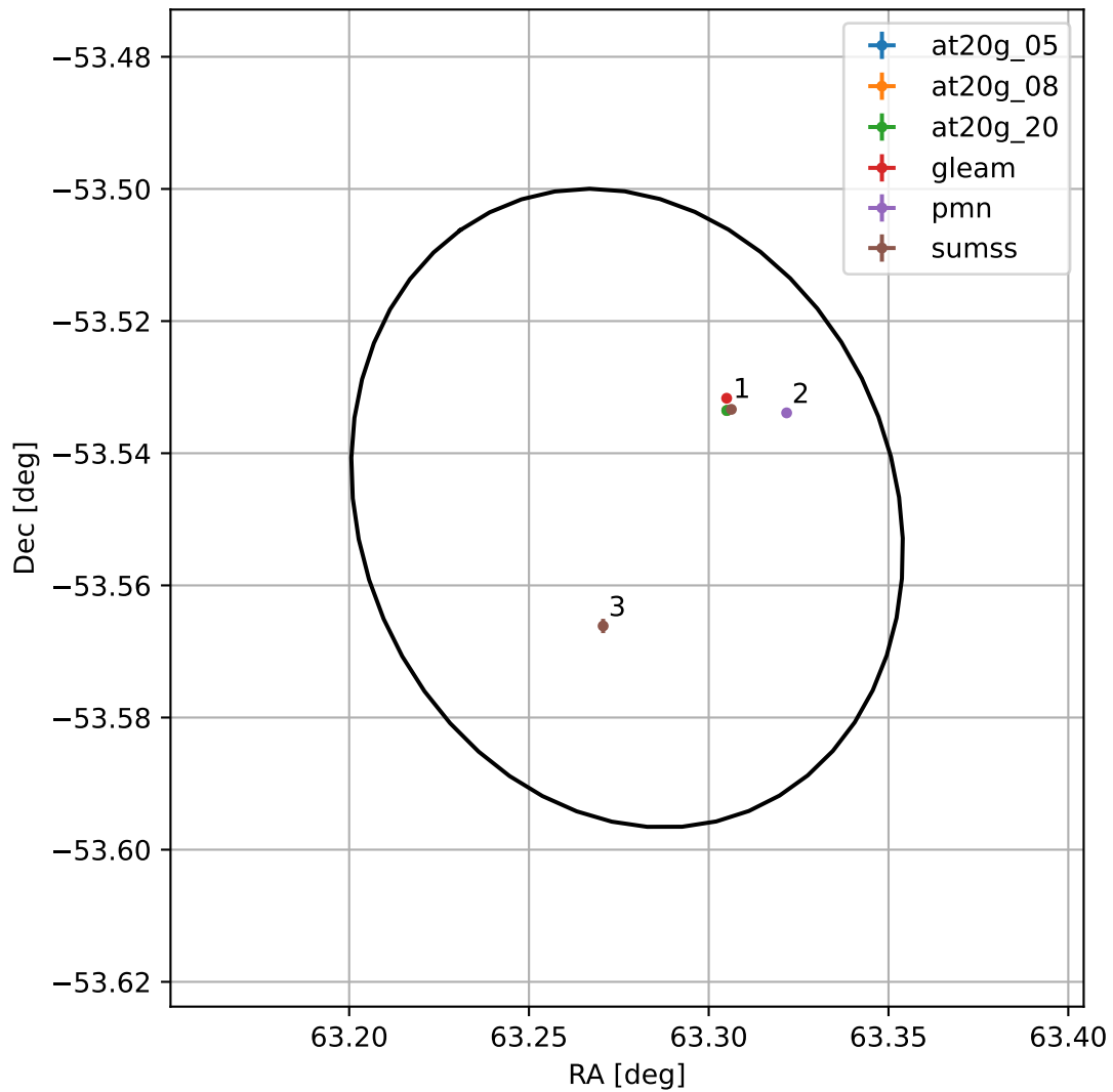
4FGL J0413.1-5332
