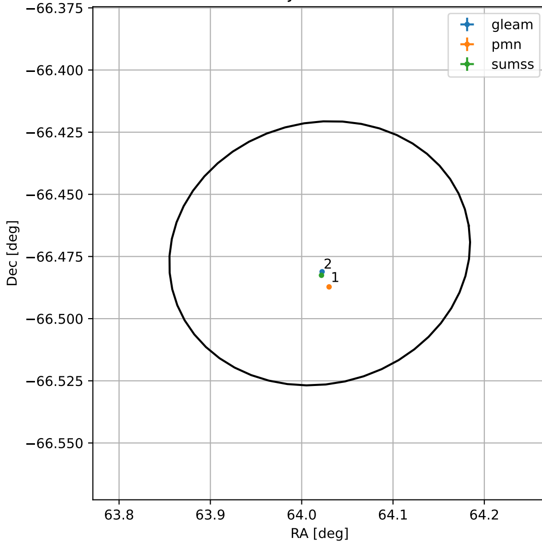
4FGL J0416.0-6628
