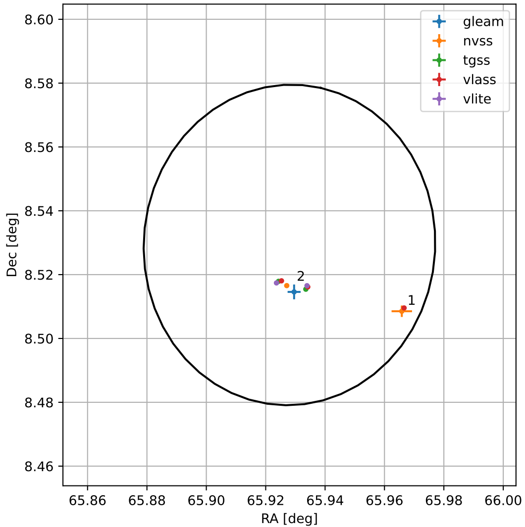
4FGL J0423.7+0831
