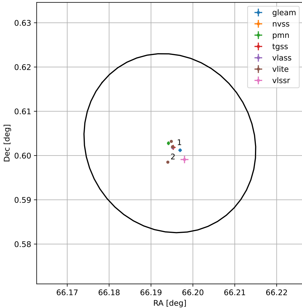
4FGL J0424.7+0036
