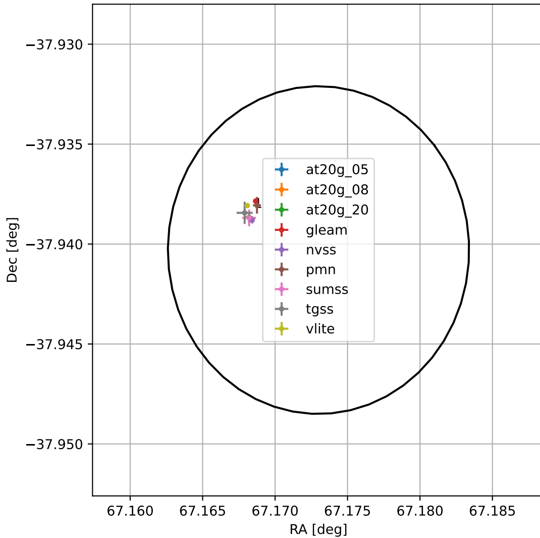
4FGL J0428.6-3756
