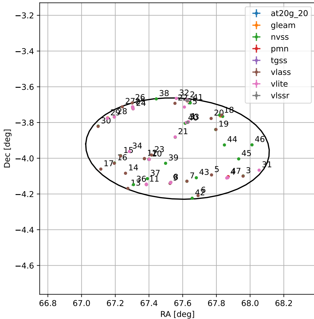
4FGL J0430.2-0356
