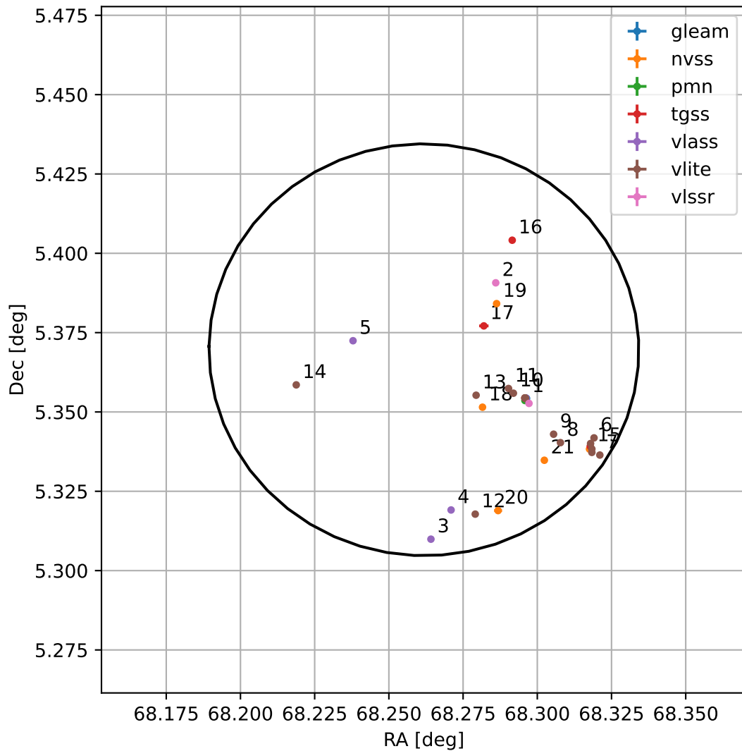
4FGL J0433.0+0522
