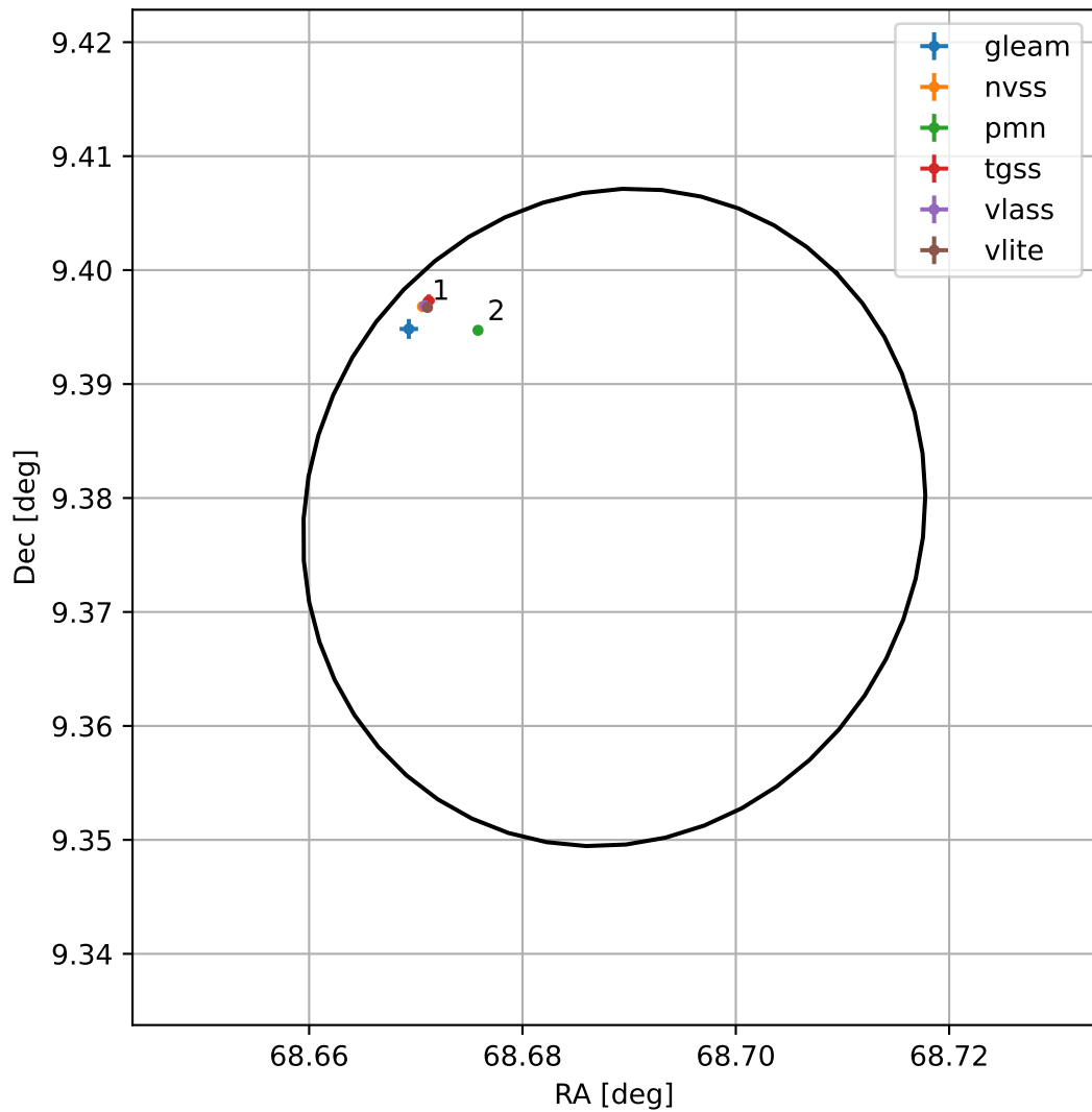
4FGL J0434.7+0922
