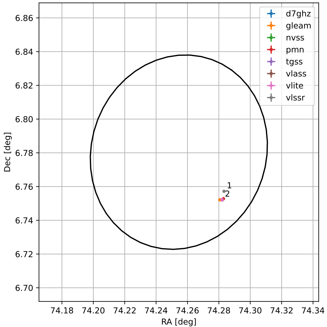
4FGL J0457.0+0646
