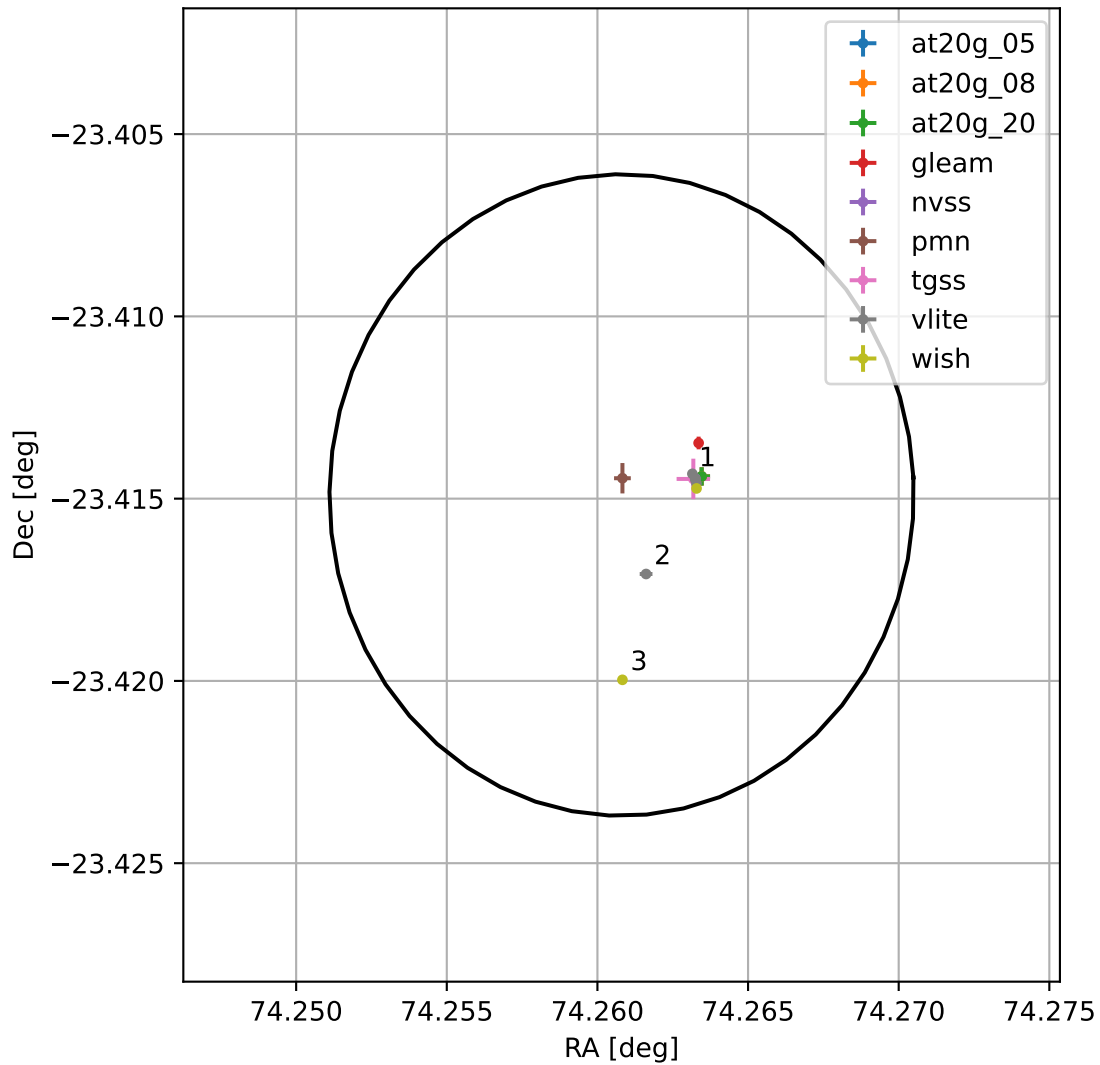
4FGL J0457.0-2324
