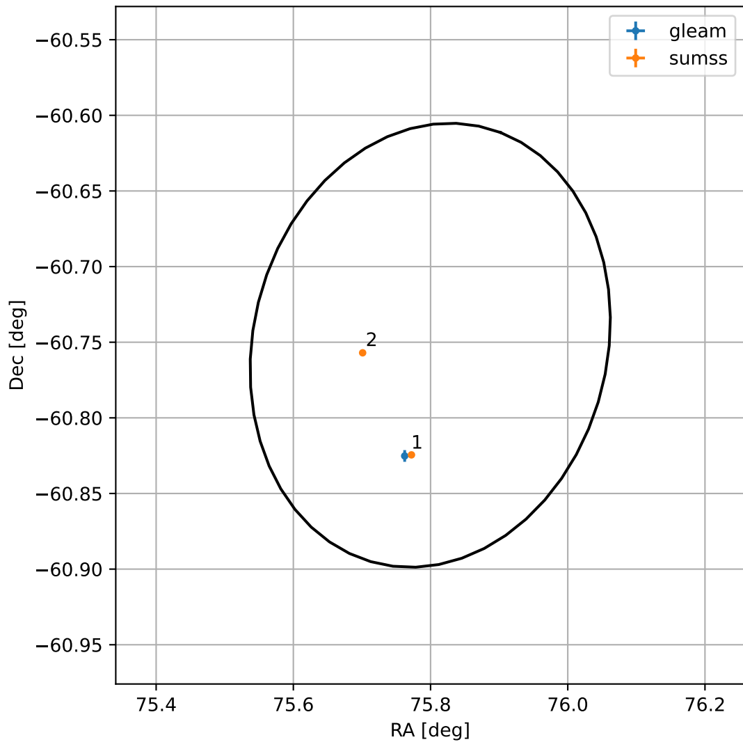
4FGL J0503.1-6045
