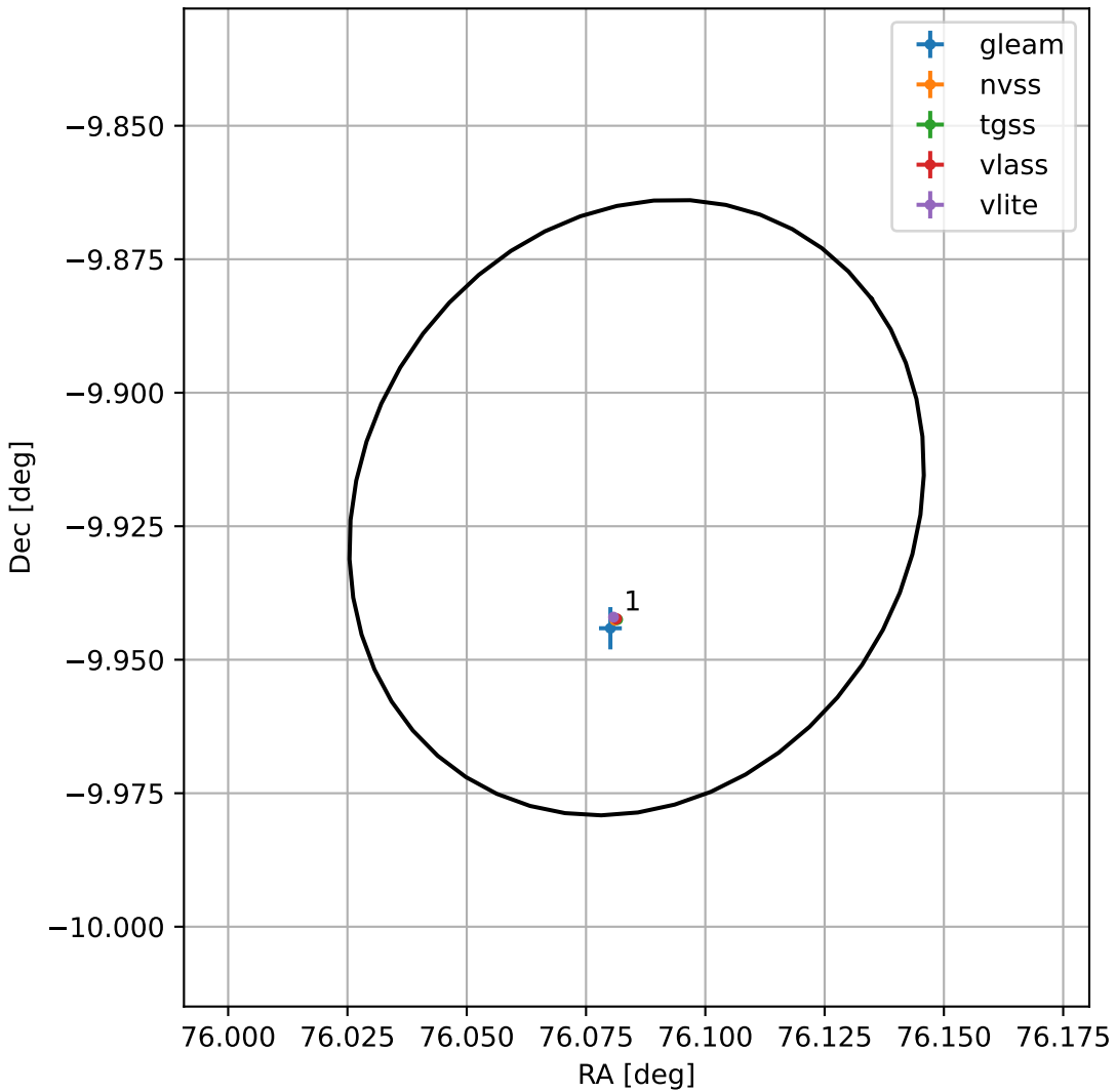
4FGL J0504.3-0955
