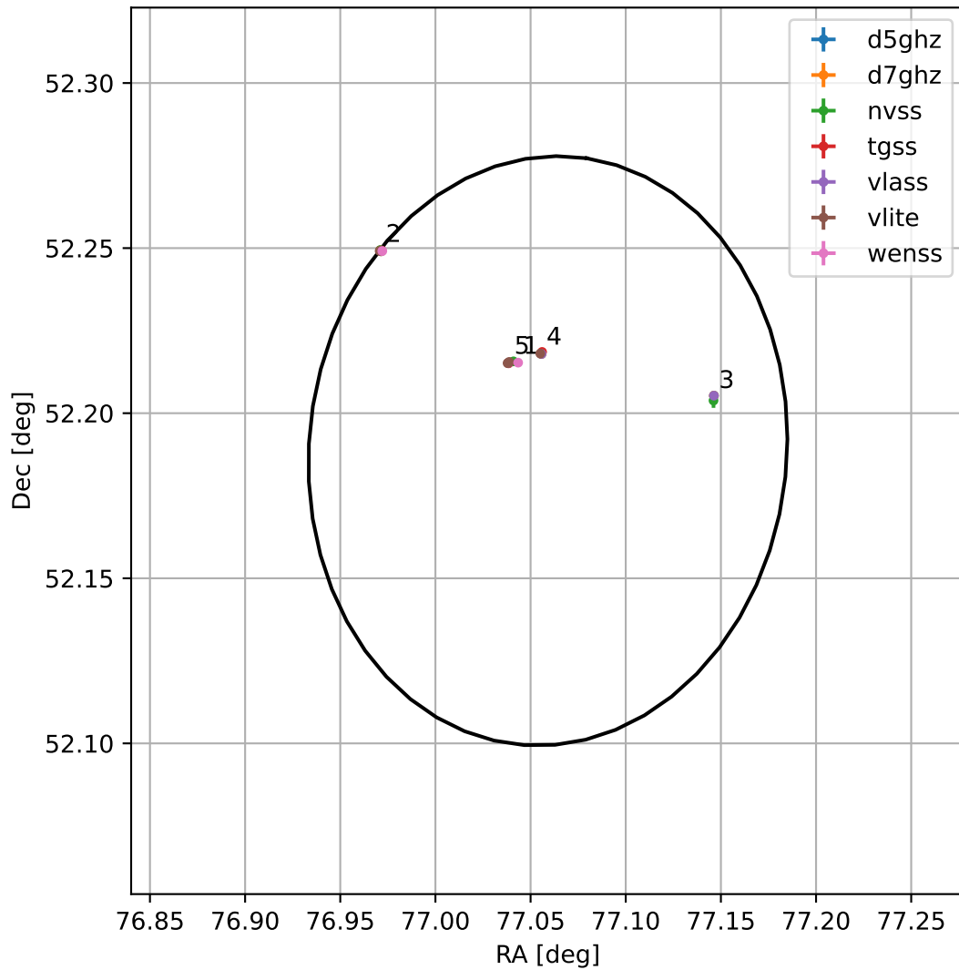
4FGL J0508.2+5211
