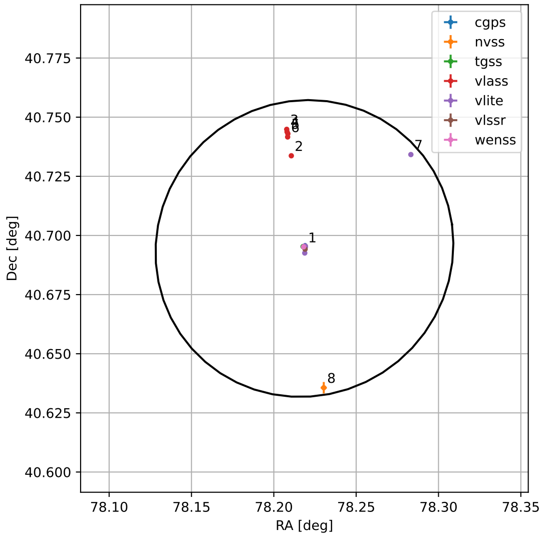
4FGL J0512.8+4041
