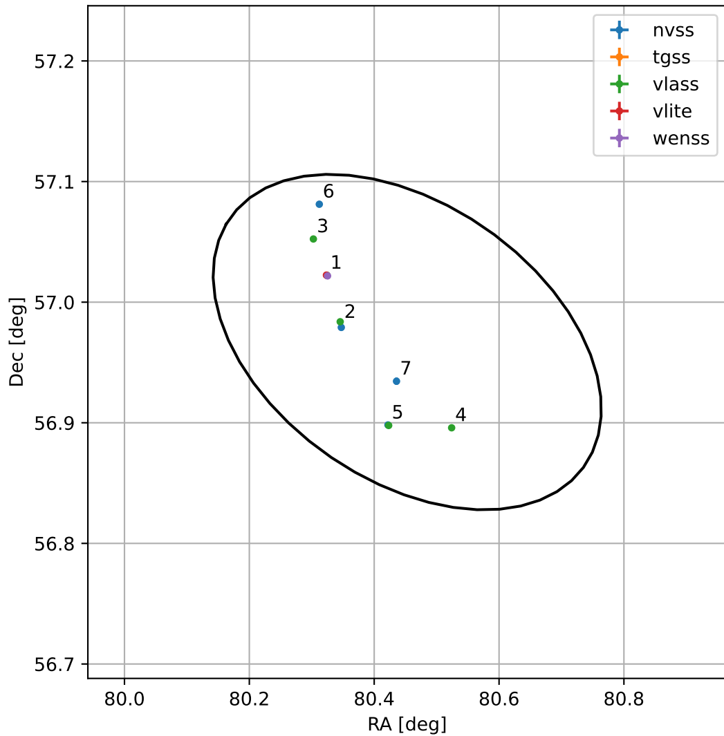
4FGL J0521.8+5658
