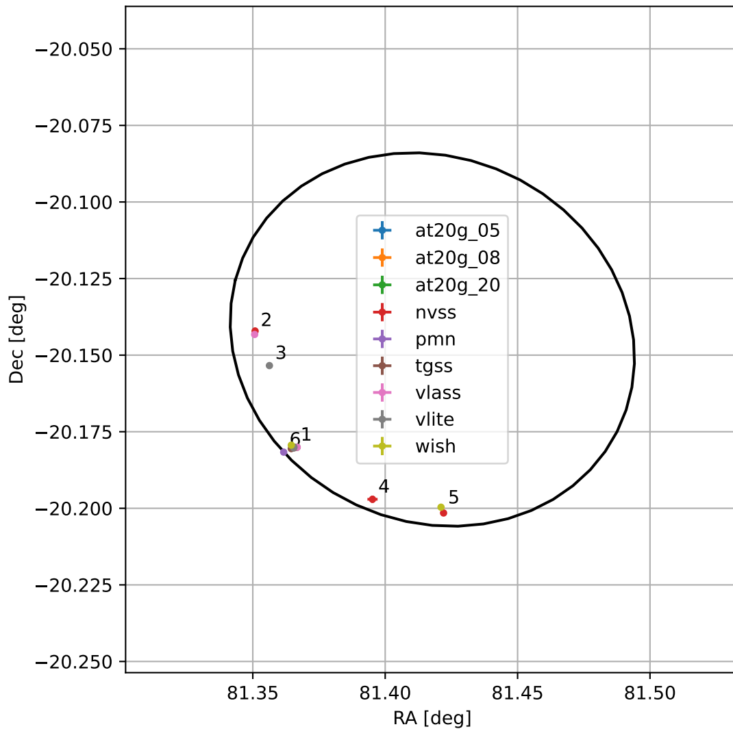
4FGL J0525.6-2008
