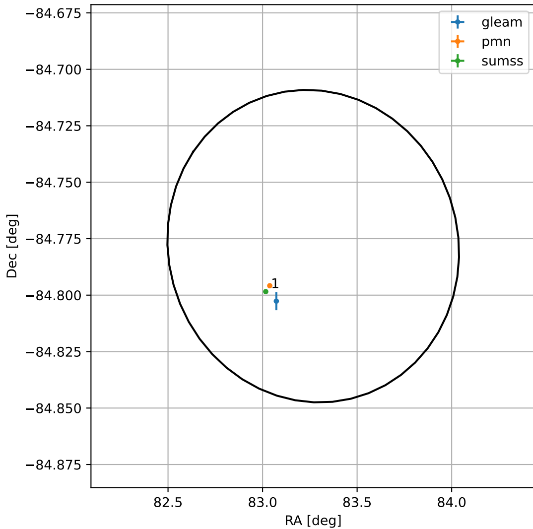
4FGL J0533.0-8446
