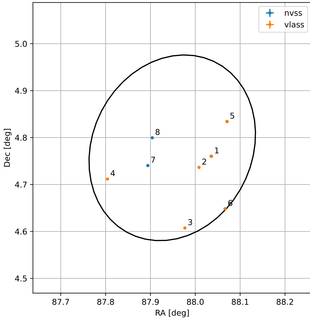
4FGL J0551.7+0446
