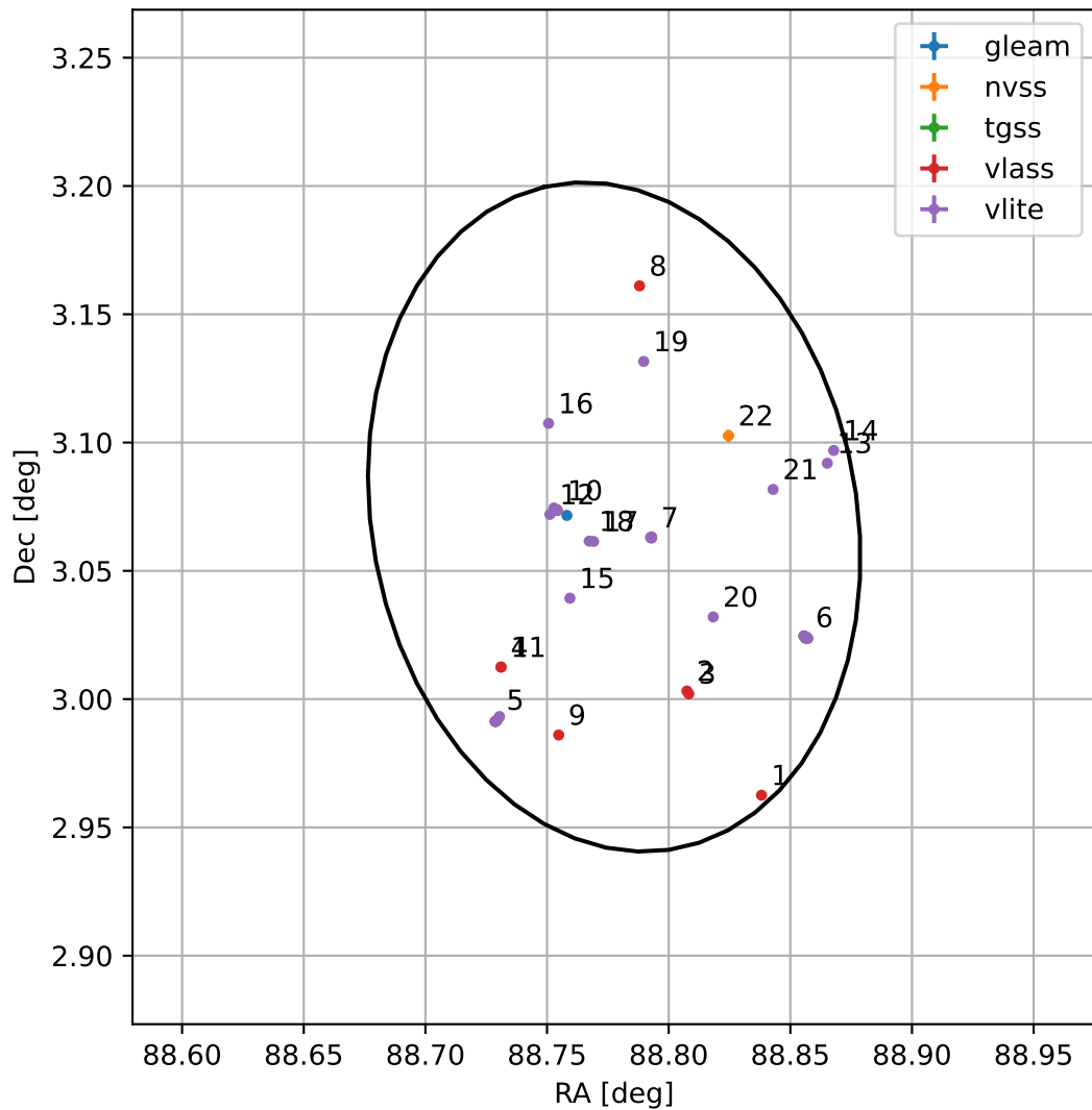
4FGL J0555.1+0304
