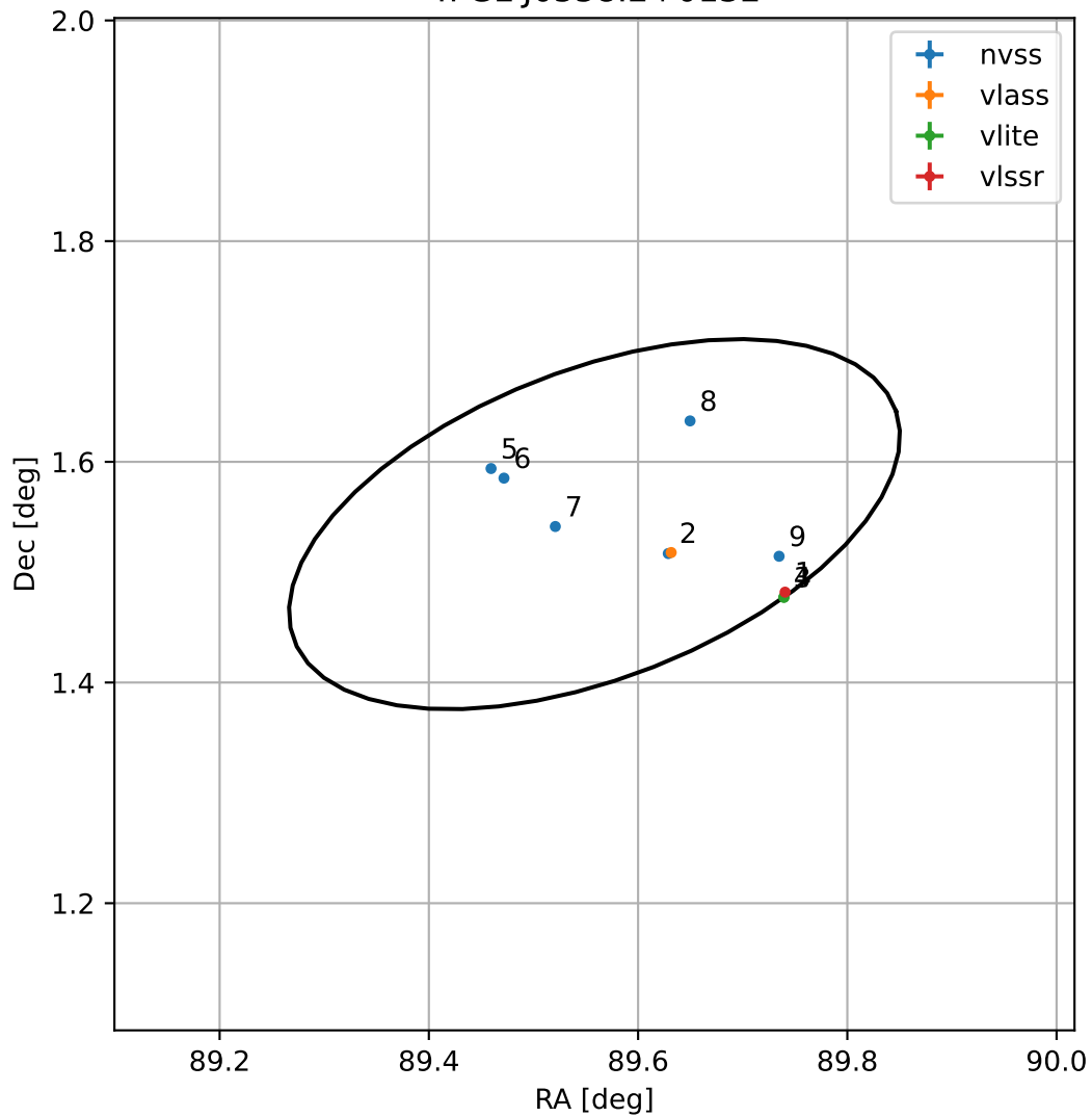
4FGL J0558.2+0132
