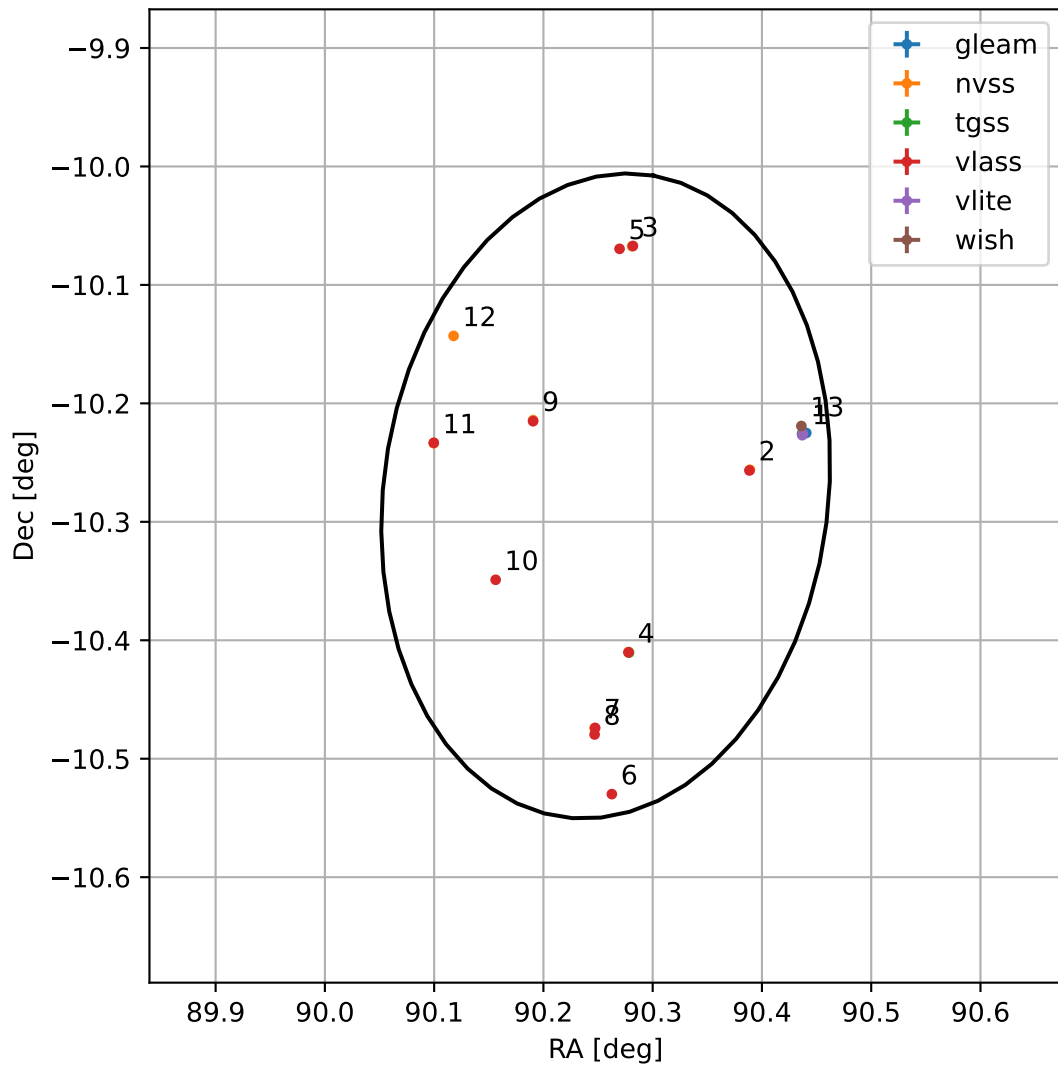
4FGL J0601.0-1016
