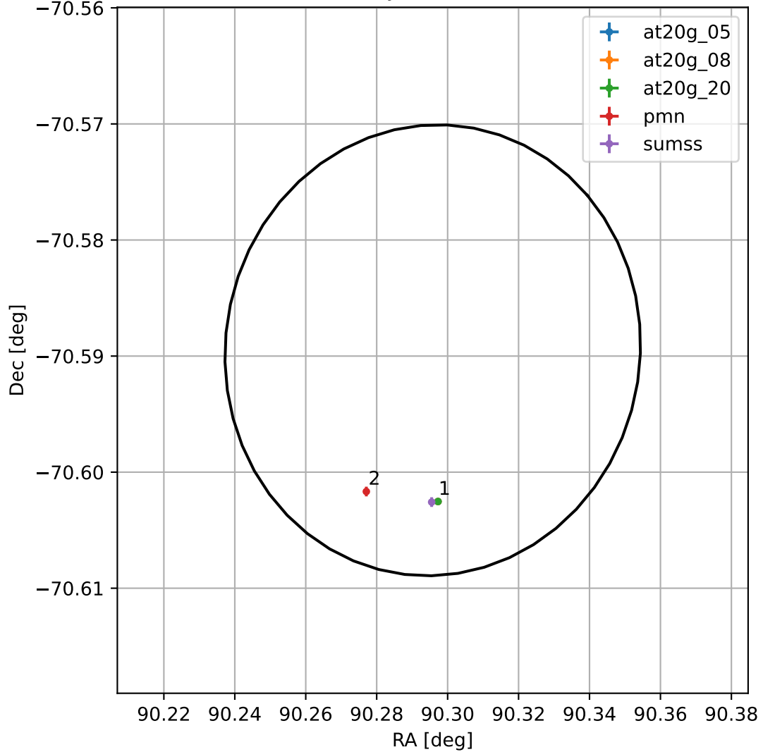
4FGL J0601.1-7035
