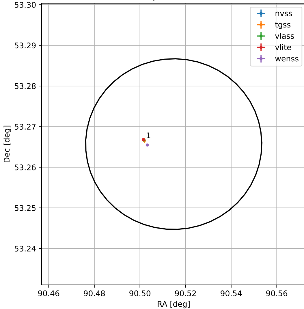
4FGL J0602.0+5315
