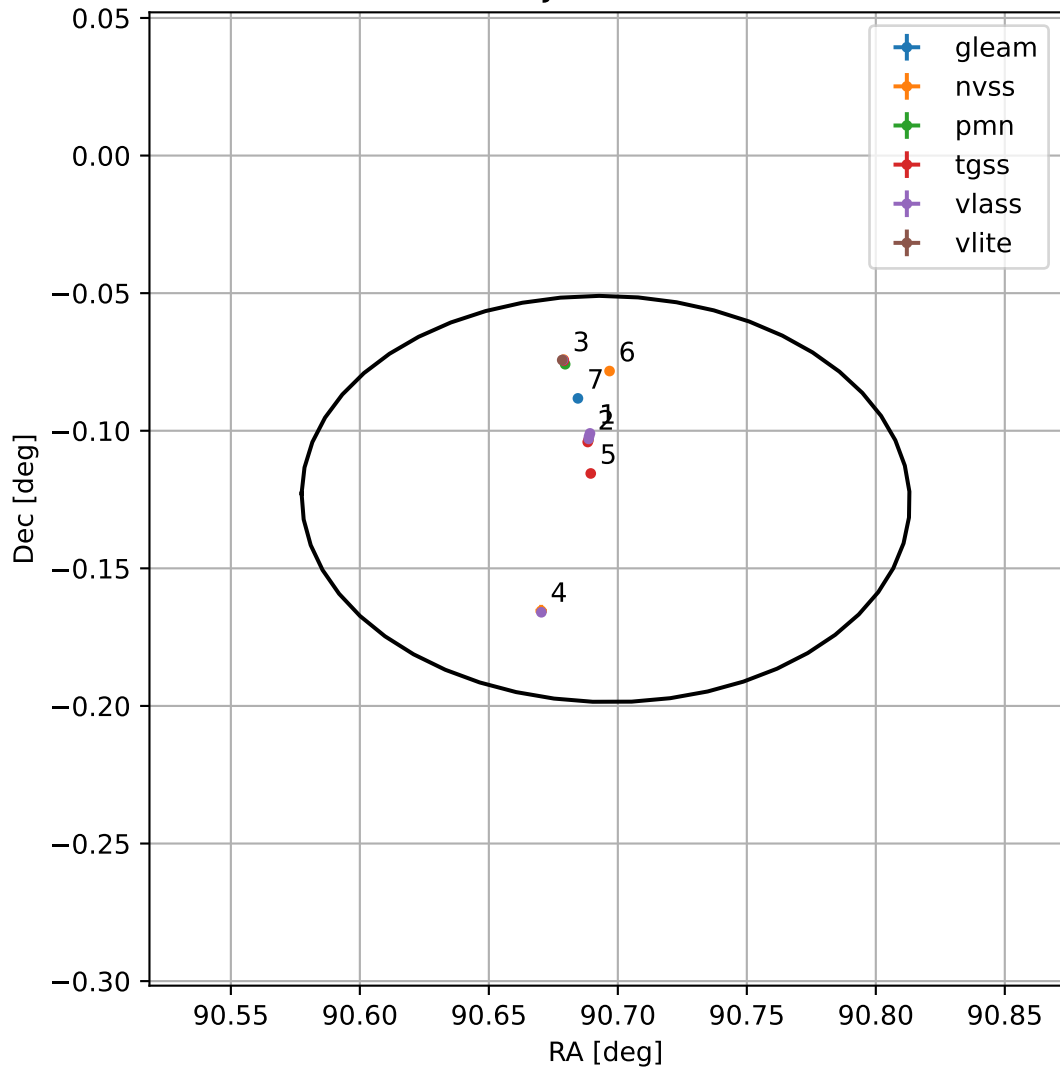
4FGL J0602.7-0007
