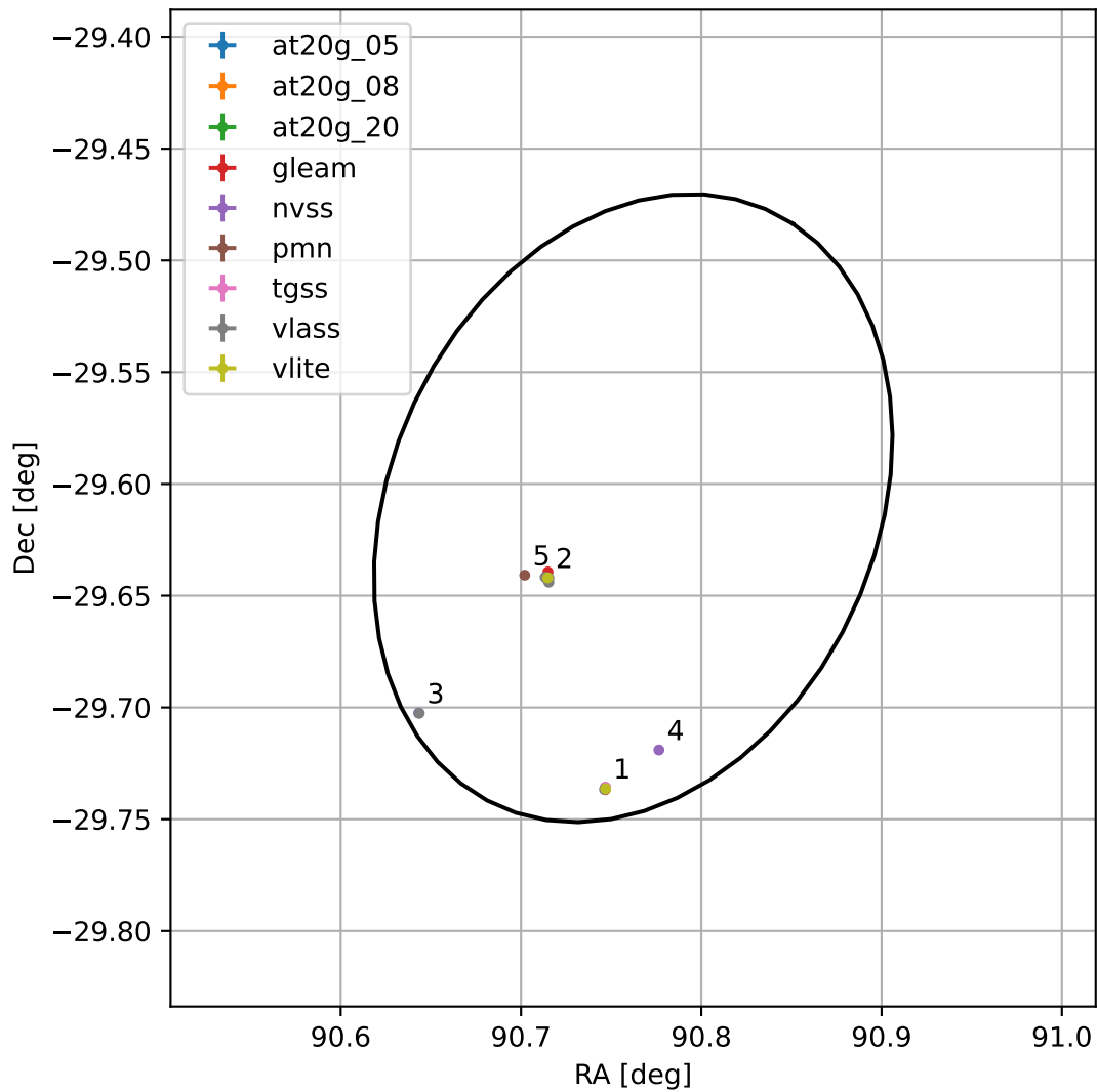
4FGL J0603.0-2936
