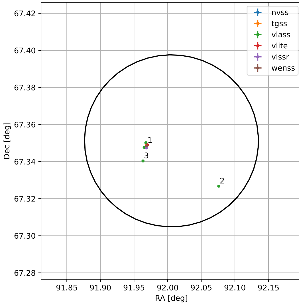
4FGL J0608.0+6721
