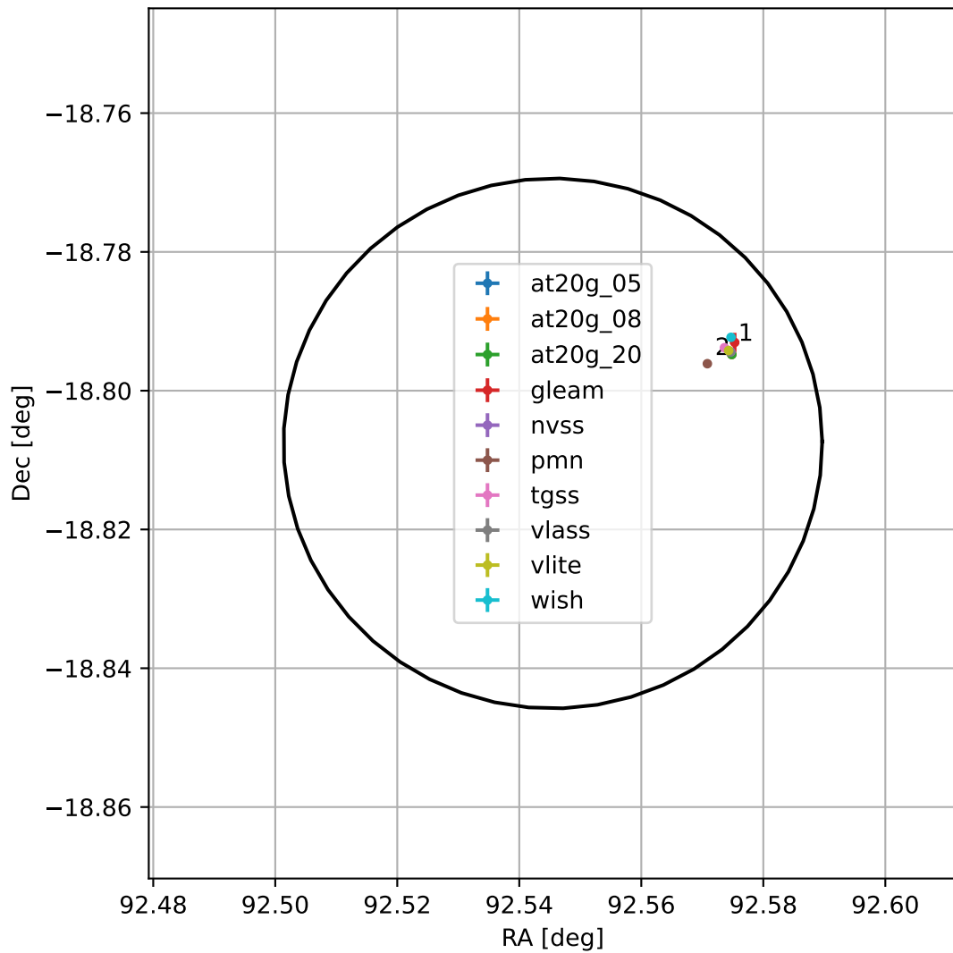
4FGL J0610.1-1848
