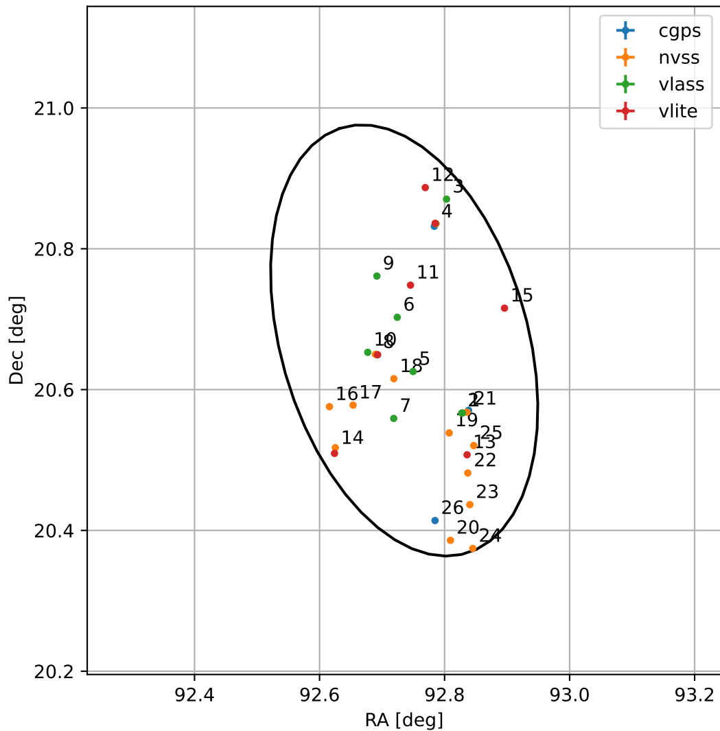
4FGL J0610.9+2040
