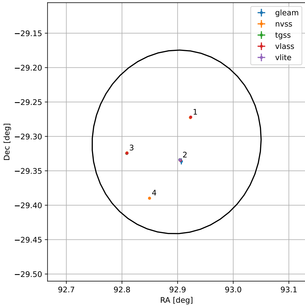
4FGL J0611.5-2918
