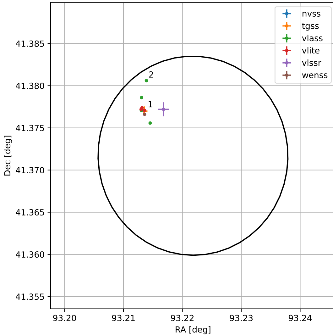
4FGL J0612.8+4122
