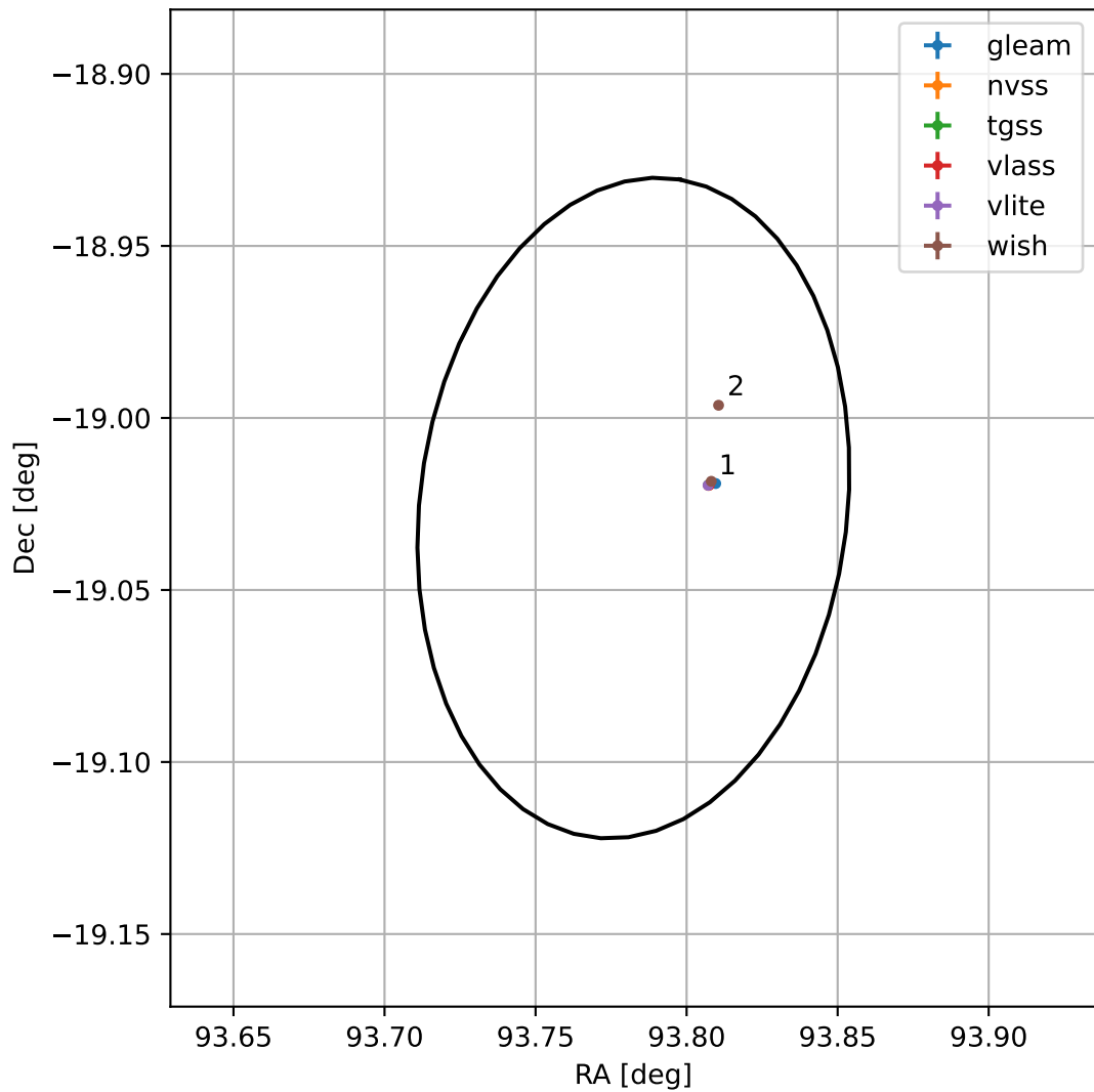
4FGL J0615.1-1901
