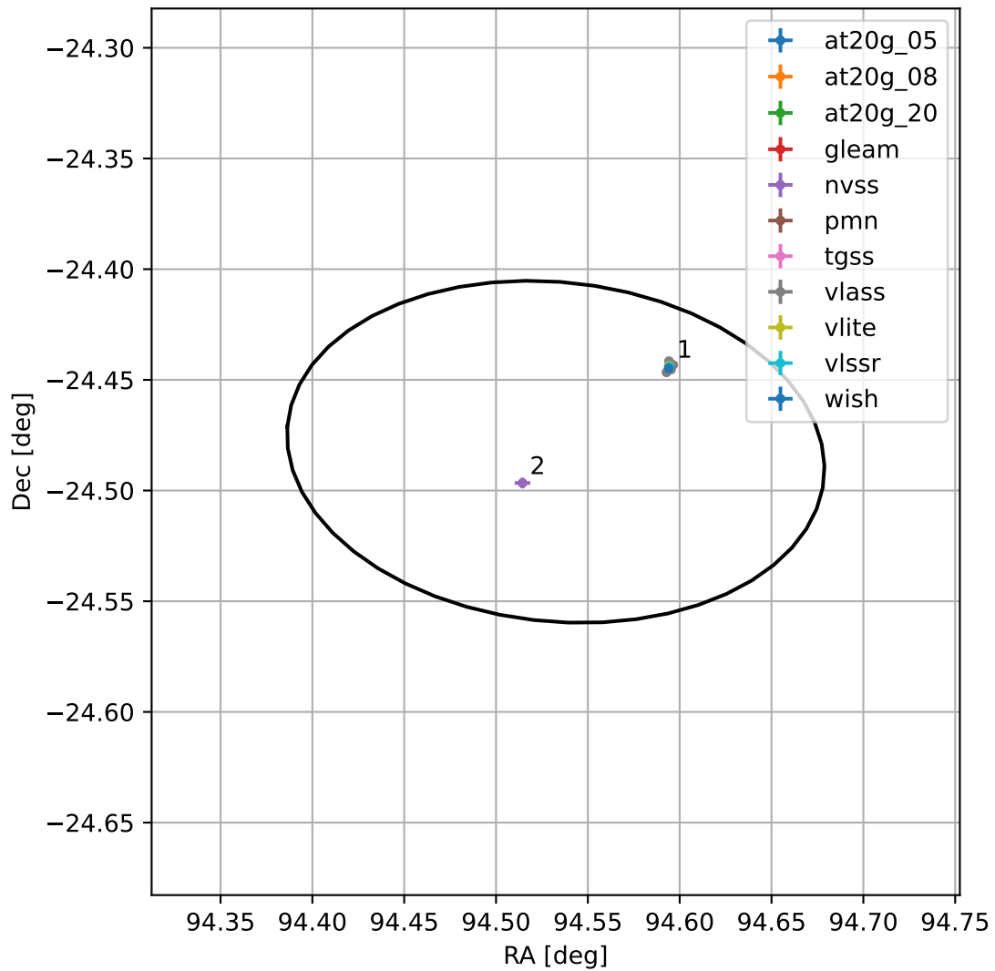
4FGL J0618.1-2428
