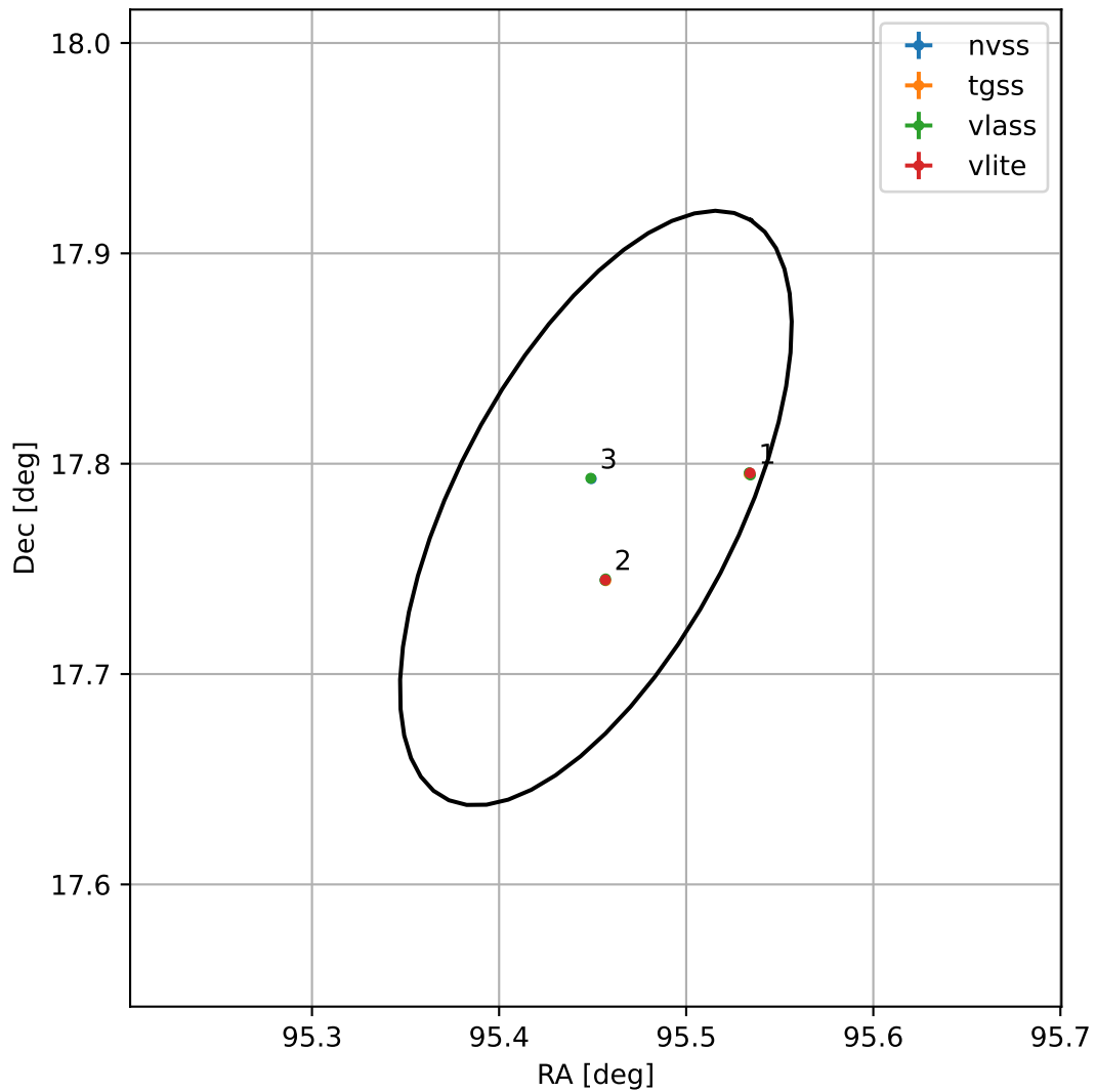
4FGL J0621.8+1746
