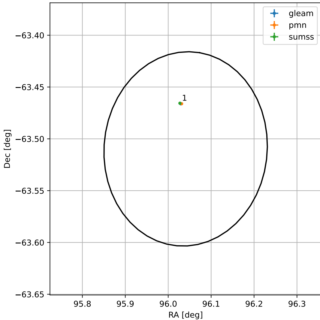
4FGL J0624.1-6330
