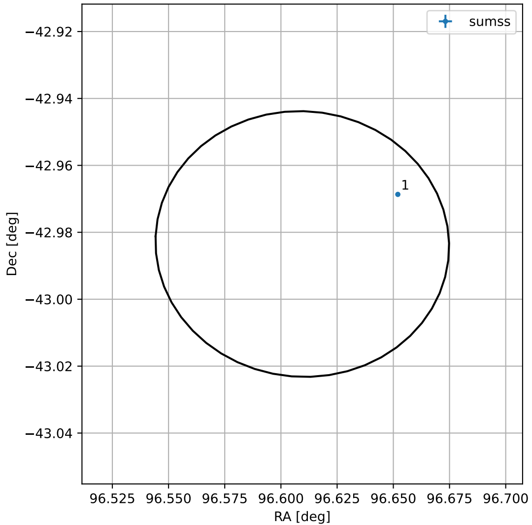
4FGL J0626.4-4259
