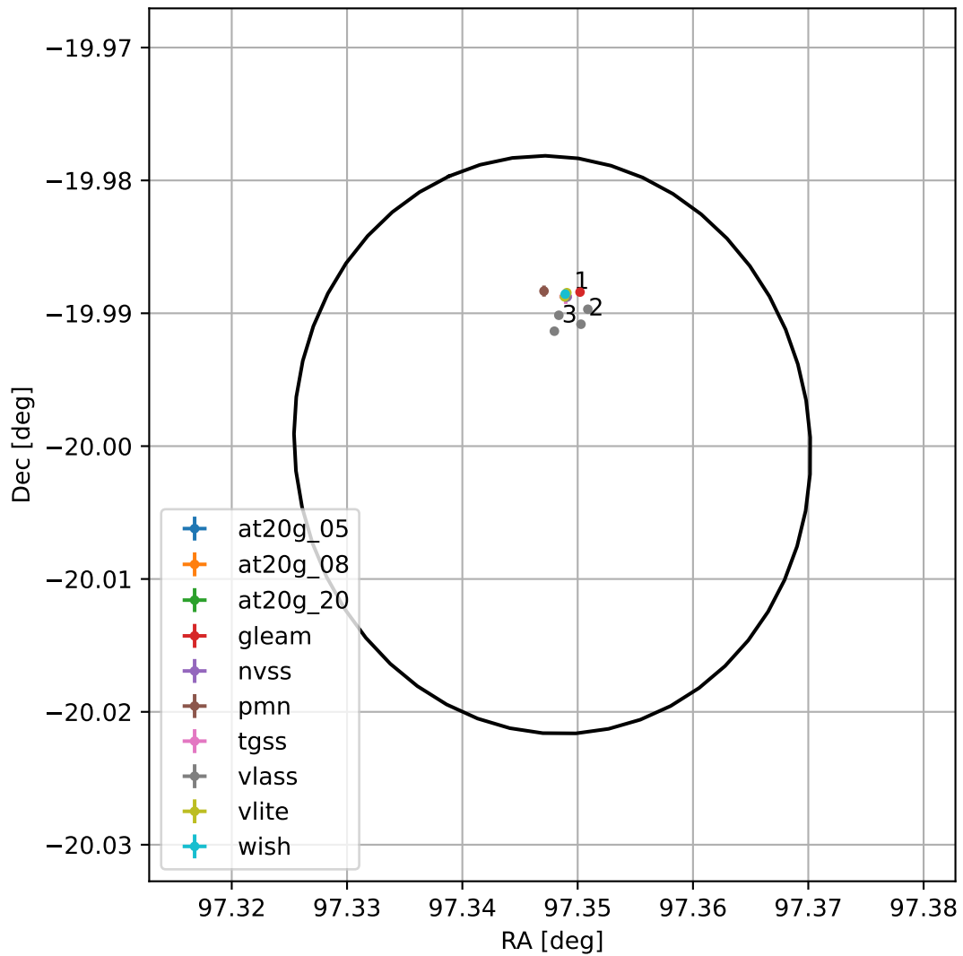
4FGL J0629.3-1959
