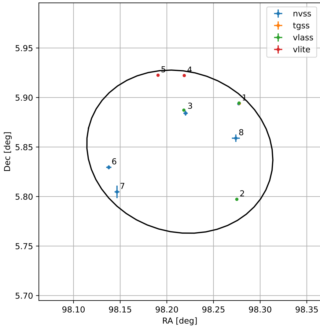
4FGL J0632.8+0550
