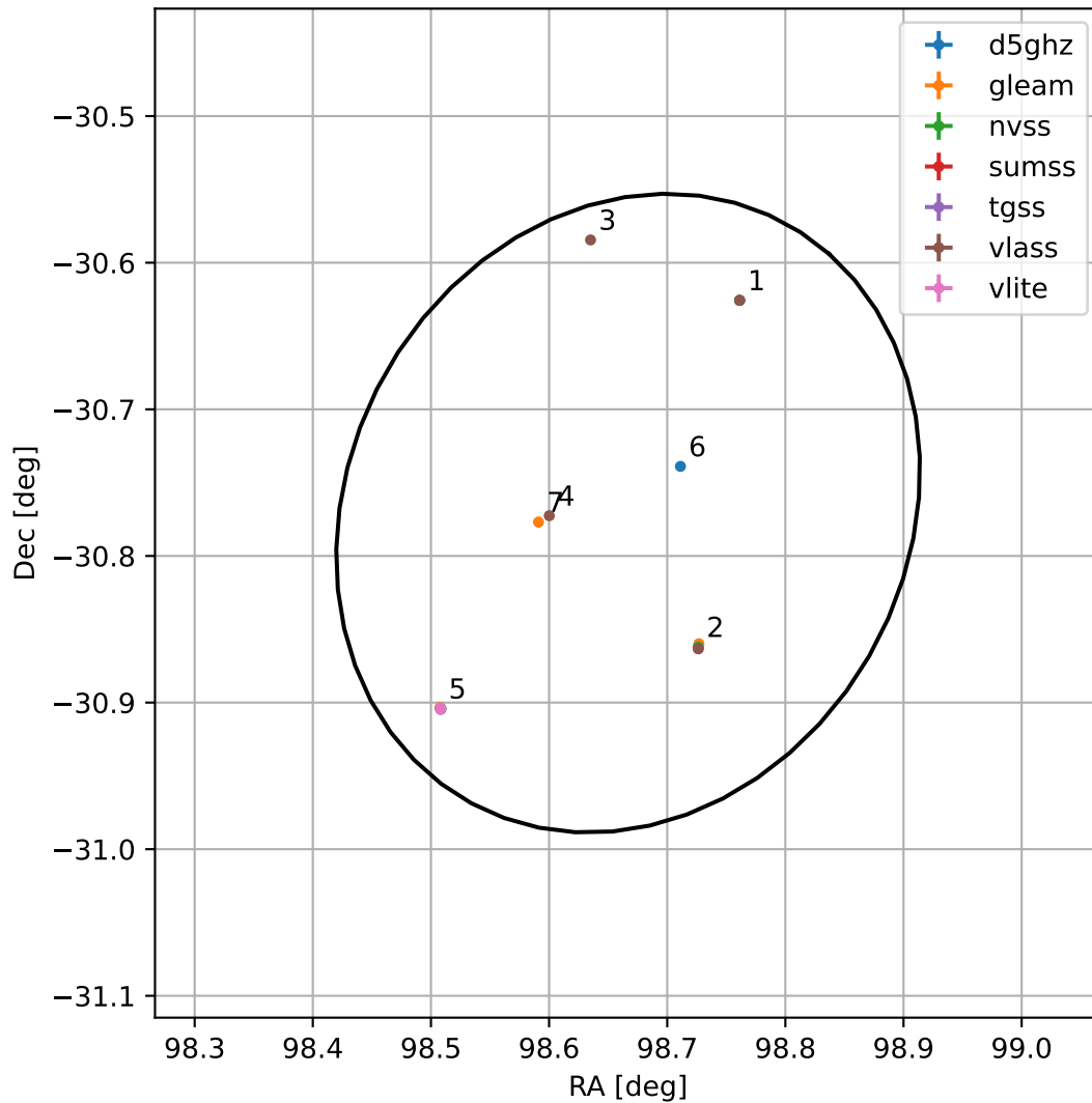
4FGL J0634.6-3046
