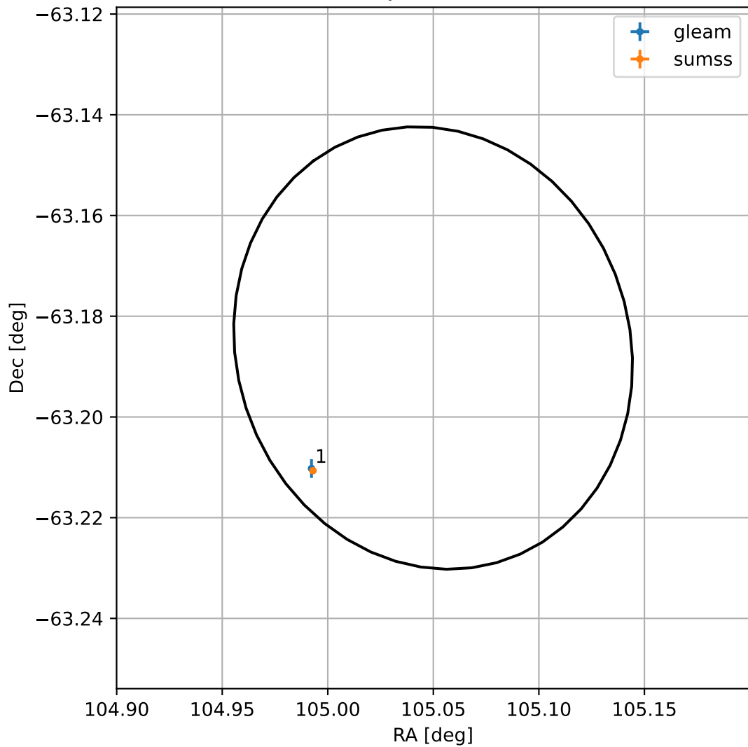
4FGL J0700.1-6311
