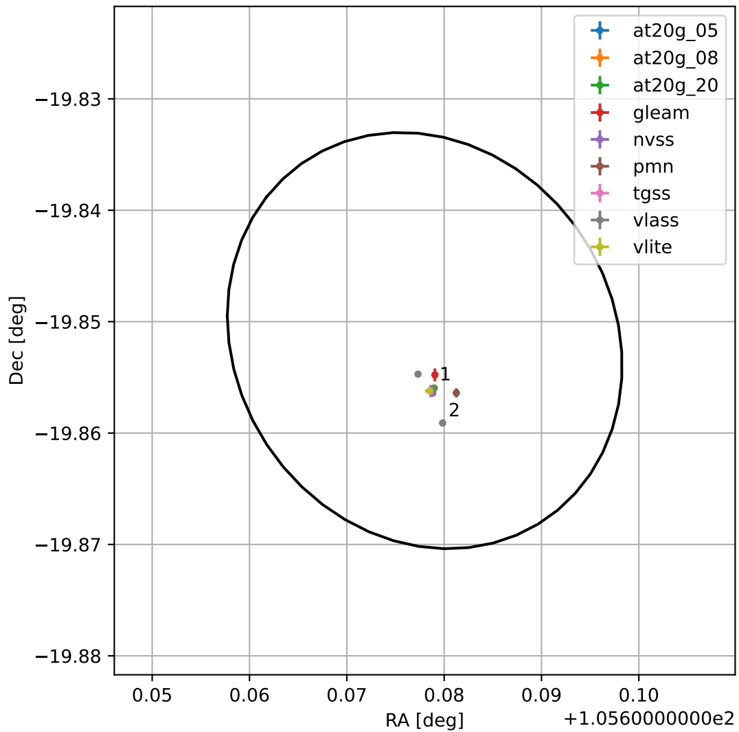
4FGL J0702.7-1951
