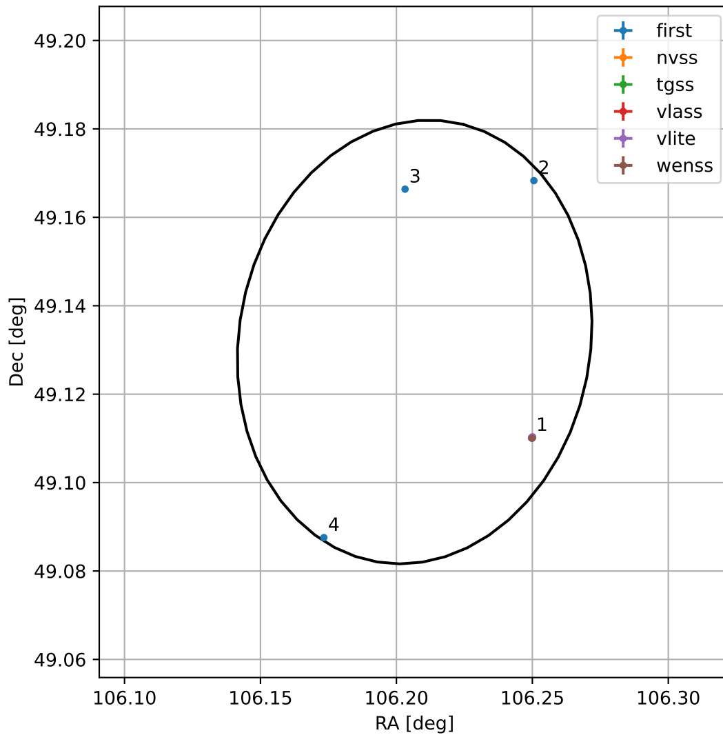
4FGL J0704.8+4907
