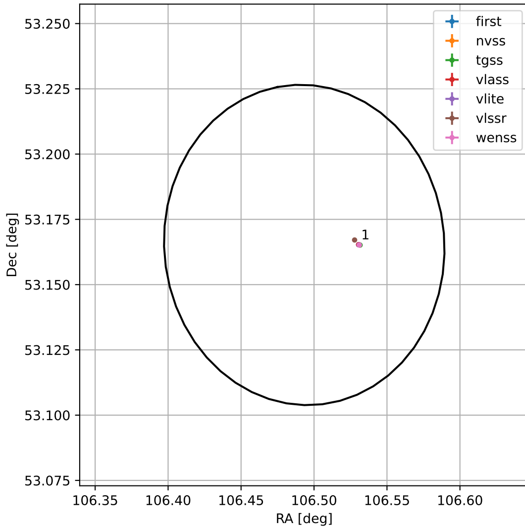
4FGL J0705.9+5309
