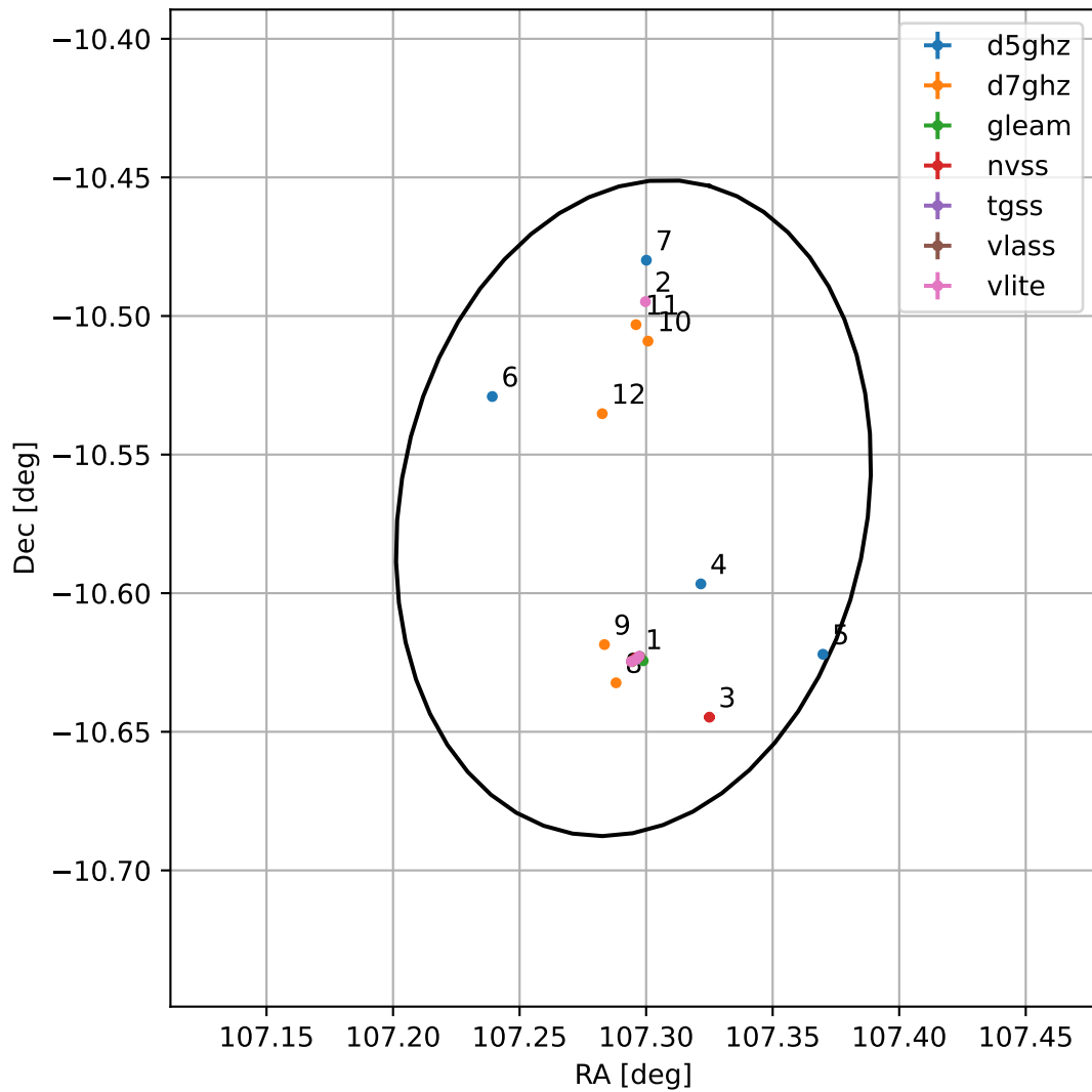
4FGL J0709.1-1034
