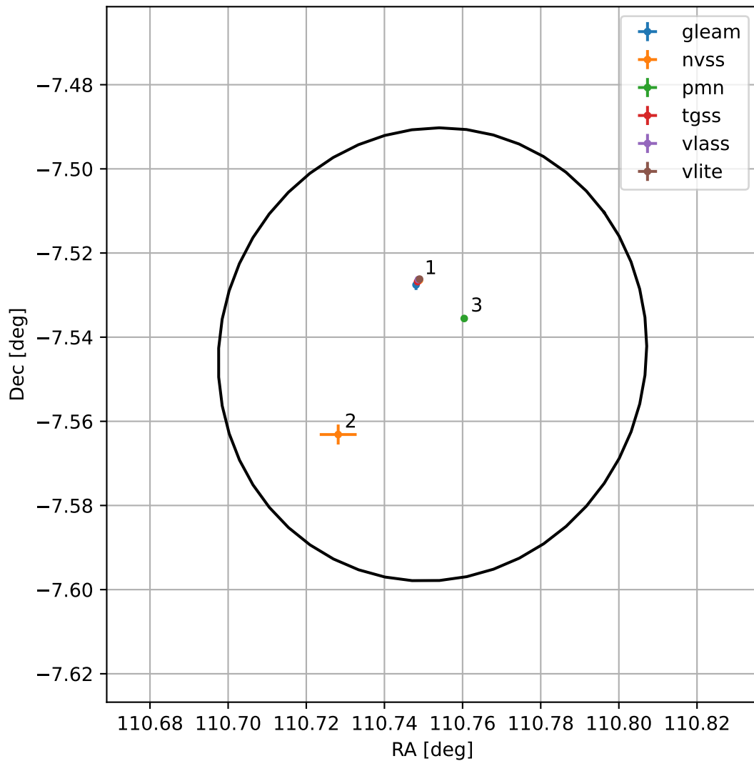
4FGL J0723.0-0732
