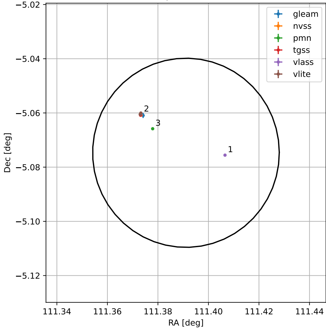
4FGL J0725.5-0504
