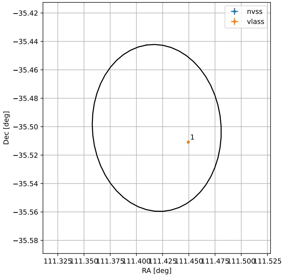
4FGL J0725.6-3530
